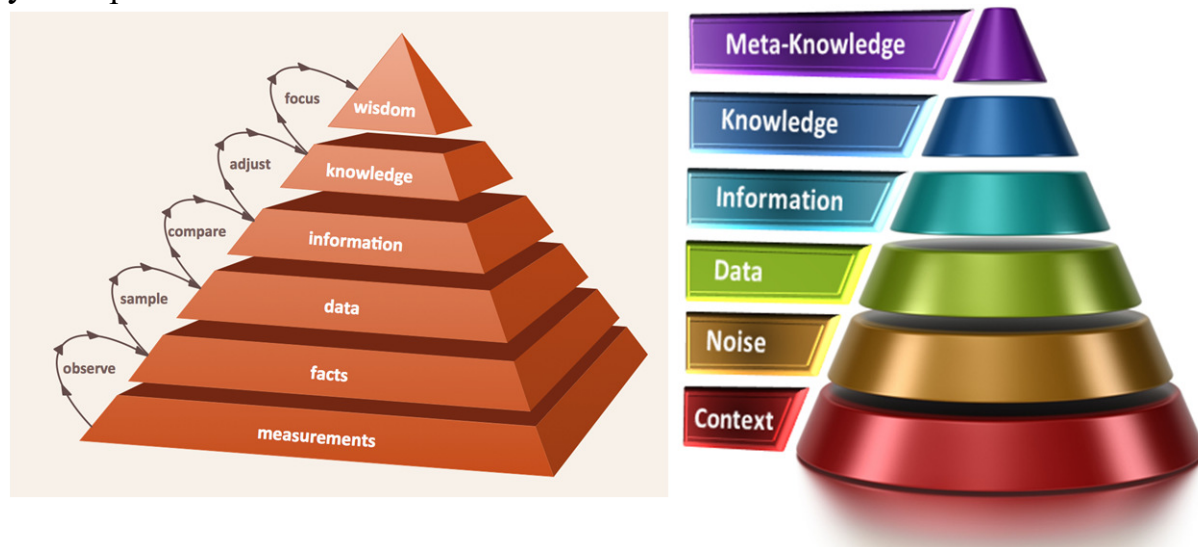
Рис. 1. Иерархия Знания
